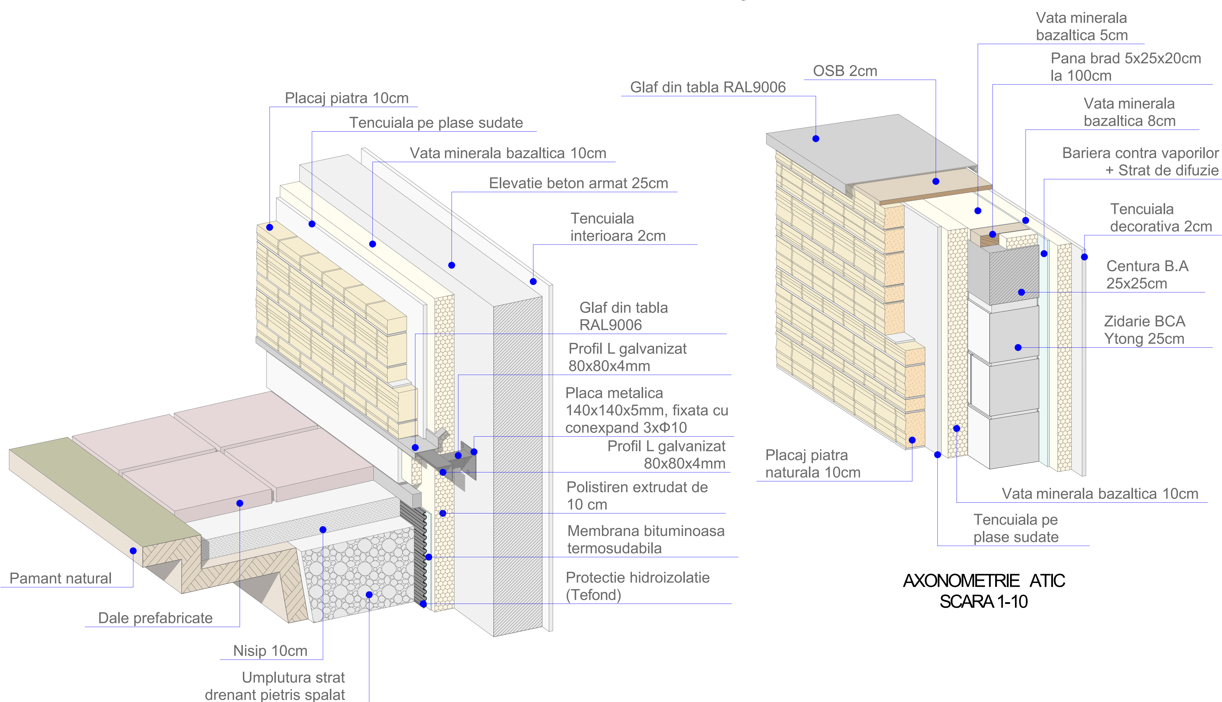
AXONOMETRIE SISTEM SUSTINERE PLACAJ PIATRA NATURALA SCARA 1-10
